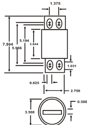
Fig. 2: 900-1000 Amp Range
