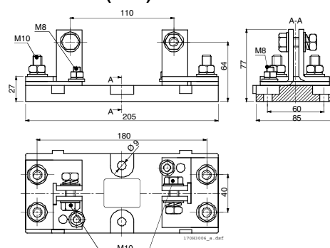
170H 3006 (IP00)
